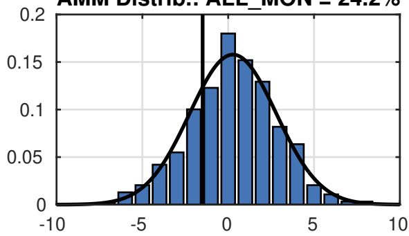
AMM Distrib.: ALL_MON = 24.2%
