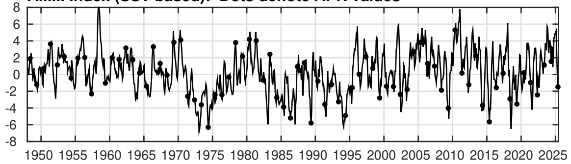
AMM Distrib.: ALL_MON = 24.2%
